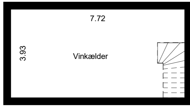
Kælderplan
